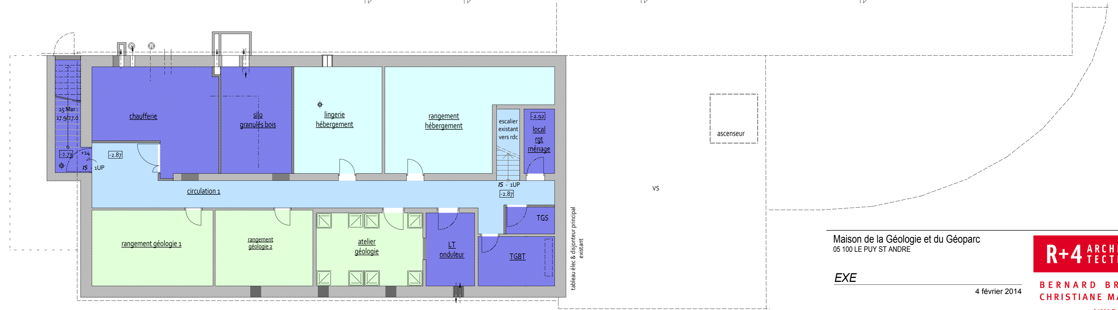
Plan - sous-sol
