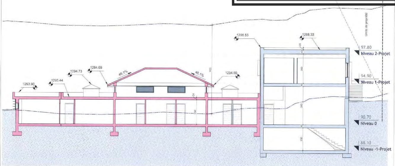
1 Coupe A 1 : 100
