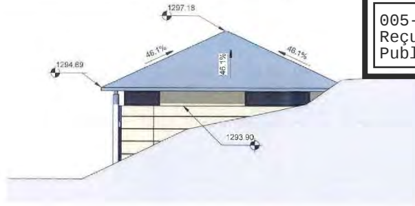
1 Façade Est - Existant 1 : 100
