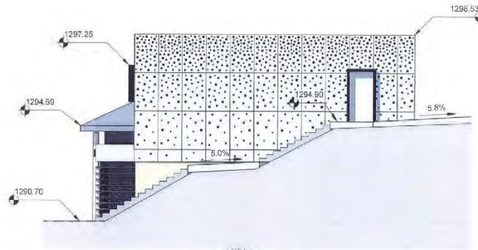
2 Façade Est - Projet 1 : 100
