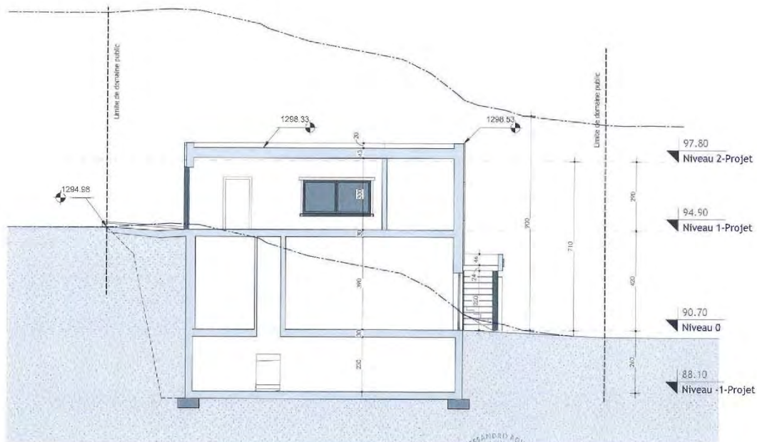
1 Section B 1 : 100
