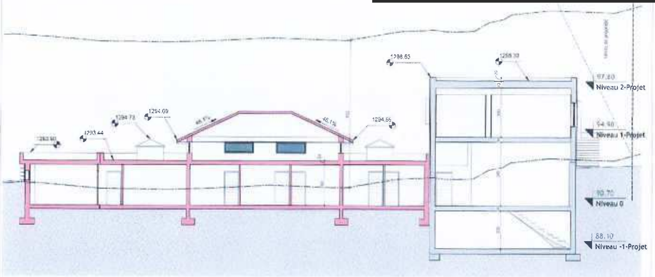
1 Coupe A 1 : 100
