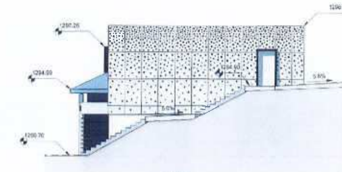
1 Façade Est - Existant 1 : 100
