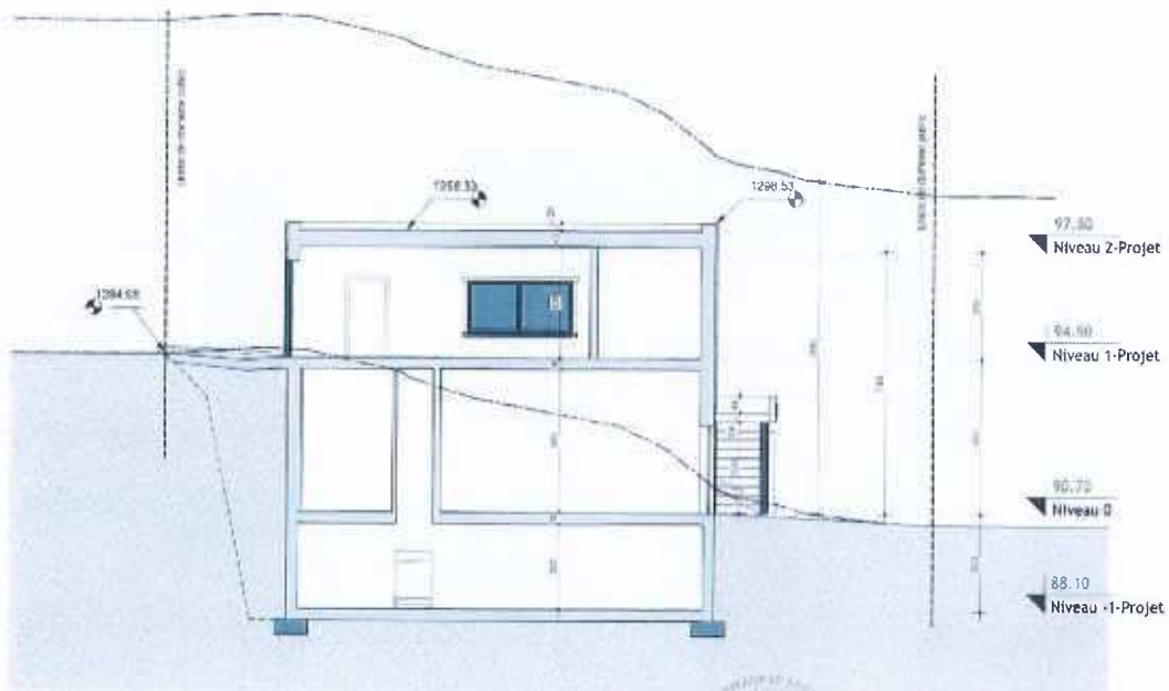
1 Section B 1 : 100
